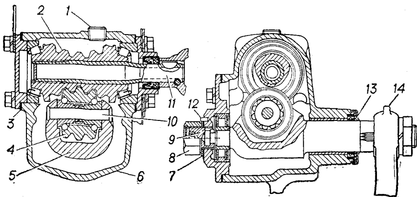
Рис. 92. Рулевой механизм:
