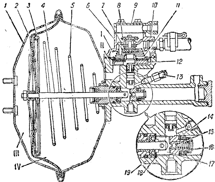
Рис. 52. Гидровакуумный усилитель:
