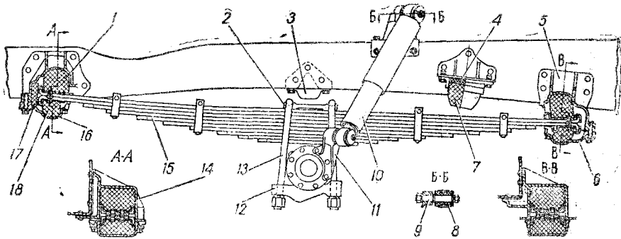
Рис. 31. Передняя подвеска
