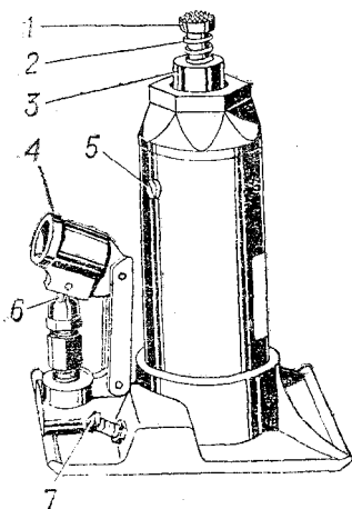
Рис. 80. Домкрат:
