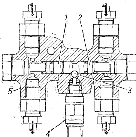
Рис. 53. Сигнальное устройство:
