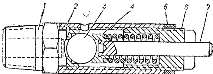
Рис. 41. Предохранительный клапан:
