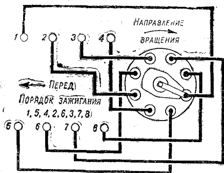
Рис. 61. Соединение проводов от датчика-распределителя к свечам
