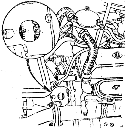
Рис. 83. Установка коленчатого вала в положение в. м. т.
