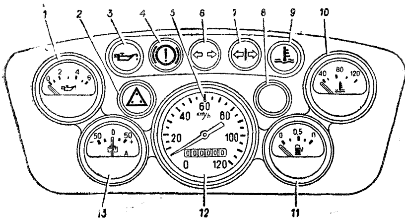
Рис. 3. Щиток приборов:
