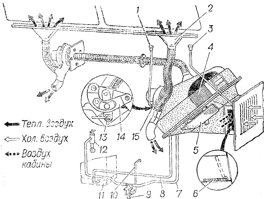
Рис. 76. Отопитель кабины:
