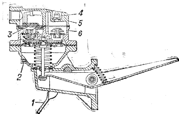
Рис. 17. Бензиновый насос:
