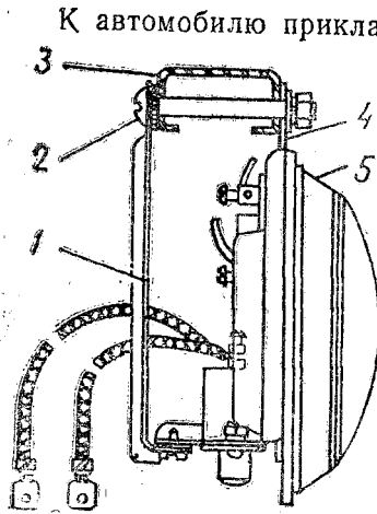
Рис. 62. Монтаж кронштейна плафона на передней дуге: 1—крышка; 2—винт; 3—дуга; 4—кронштейн; 5—плафон
