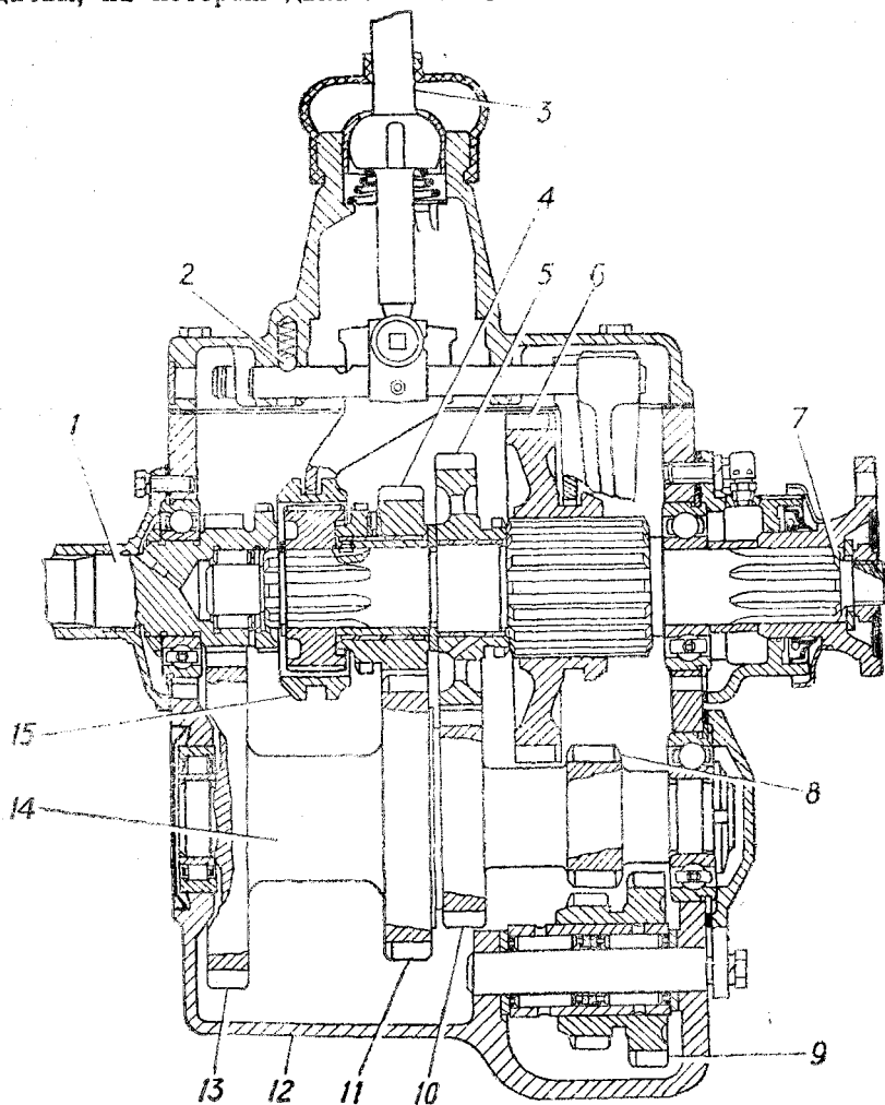
Рис. 26. Коробка передач:
